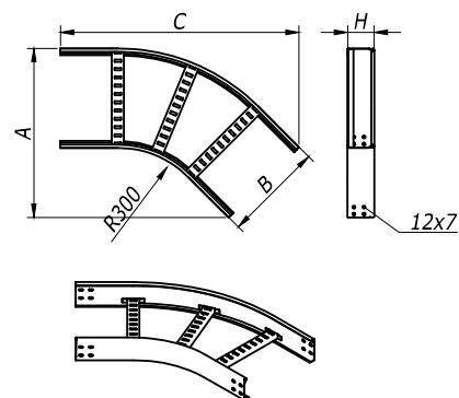
Угол горизонтальный 45° R-300
