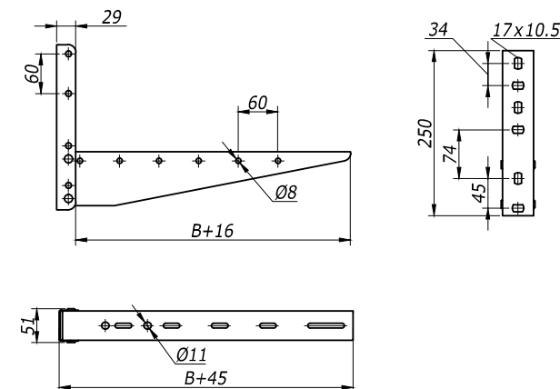
Консоль ВВЛ-55
