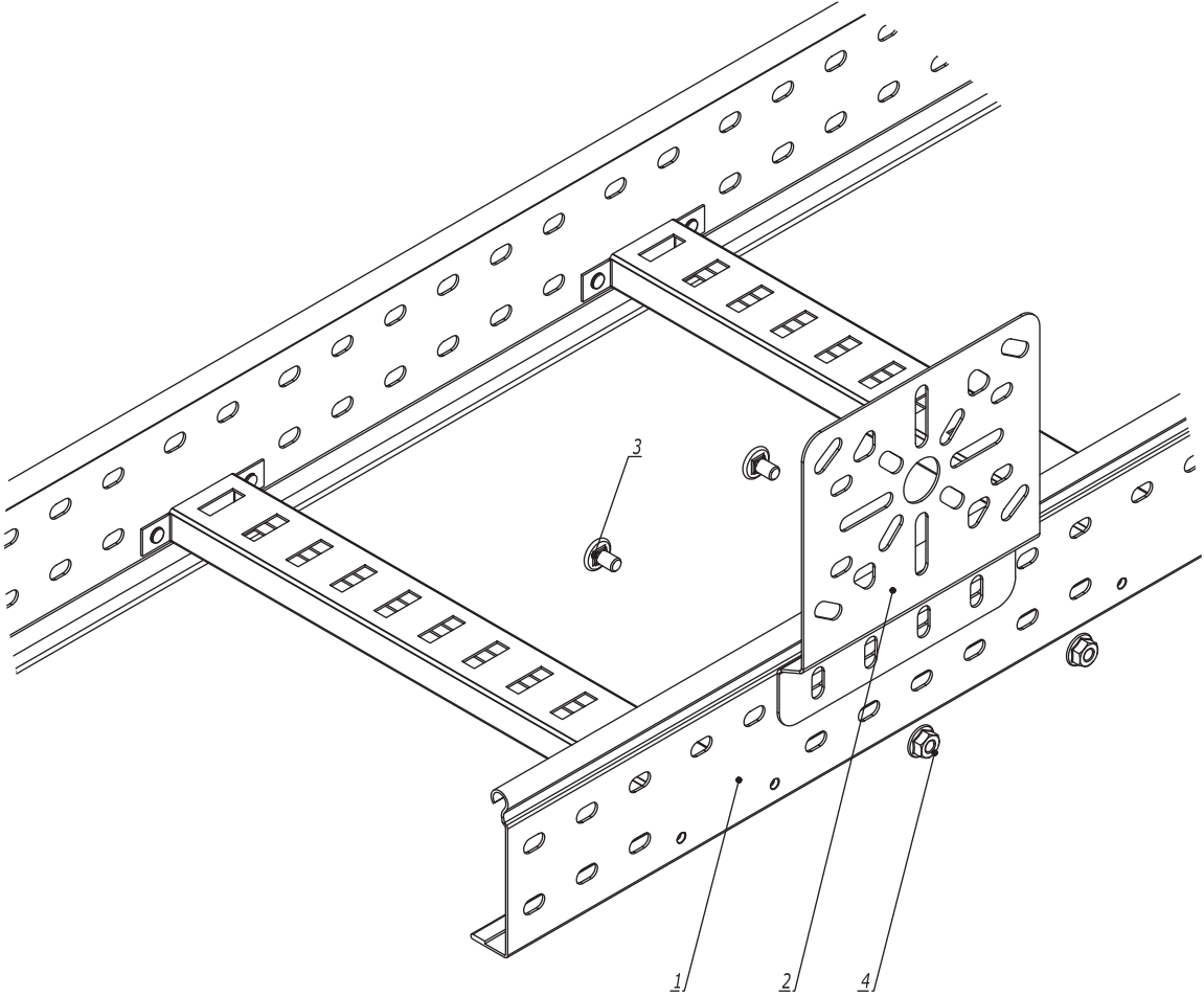
Пластина вертикальная
