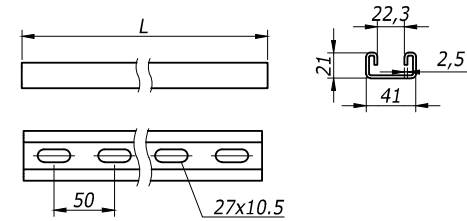
Профиль BPM-21
